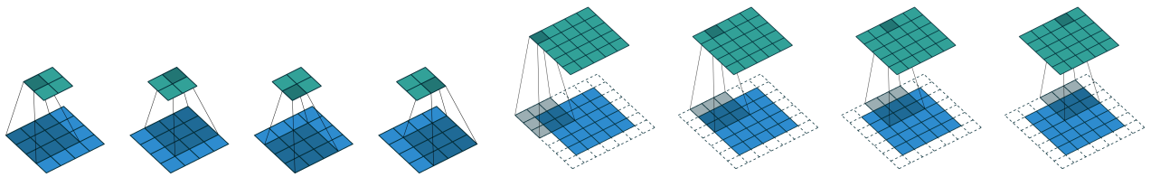
(a) Convolution simple, pas de padding, stride de 1, kernel de taille 3. (b) Convolution avec padding de 1, stride de 1, kernel de taille 3.
