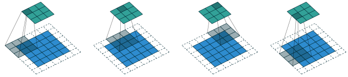
(c) Exemple de max pooling, pas de padding, stride de 2, kernel de taille 2. (d) Convolution avec padding de 1, stride de 2, kernel de taille 3.
